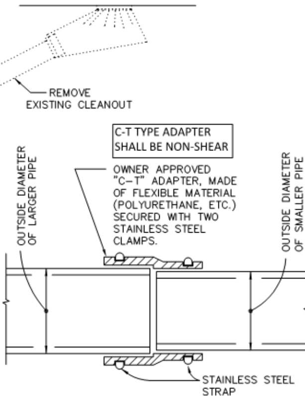
"C-T" PIPE ADAPTER N.T.S.
